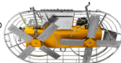
PALE CHE SI INCROCIANO OVERLAPPING BLADES
