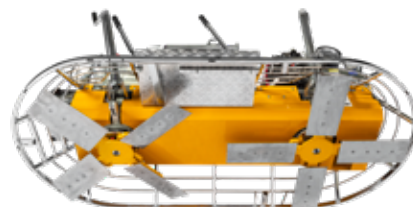
PALE CHE NON SI INCROCIANO NON-OVERLAPPING BLADES
