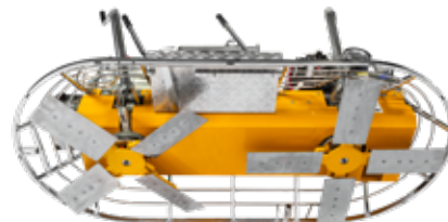
PALE CHE NON SI INCROCIANO NON-OVERLAPPING BLADES
