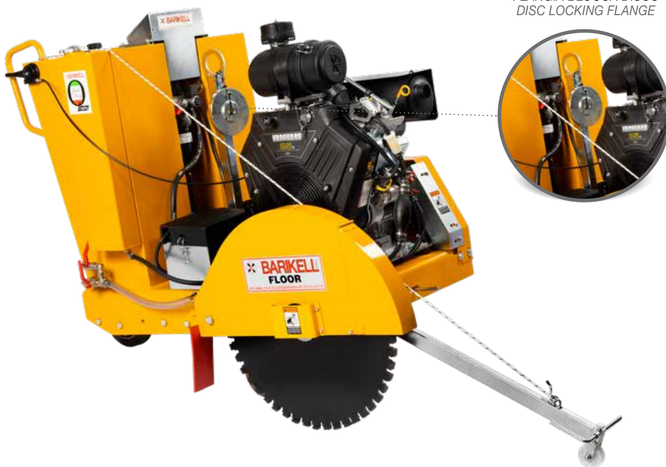
FLANGIA BLOCCA DISCO DISC LOCKING FLANGE
